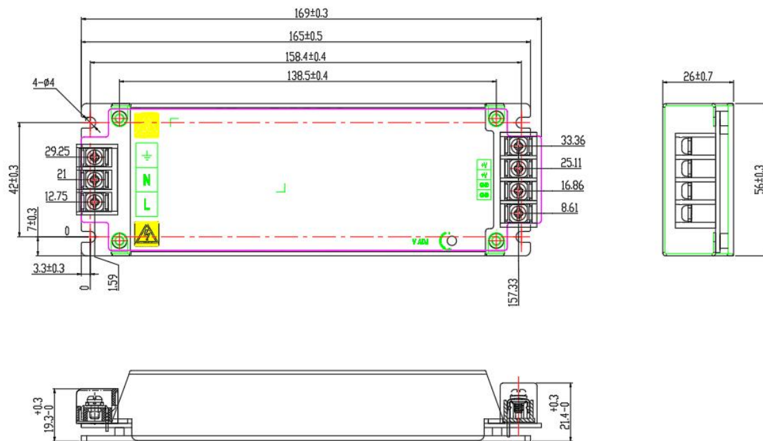
外形尺寸及安装孔——端子坐标图
